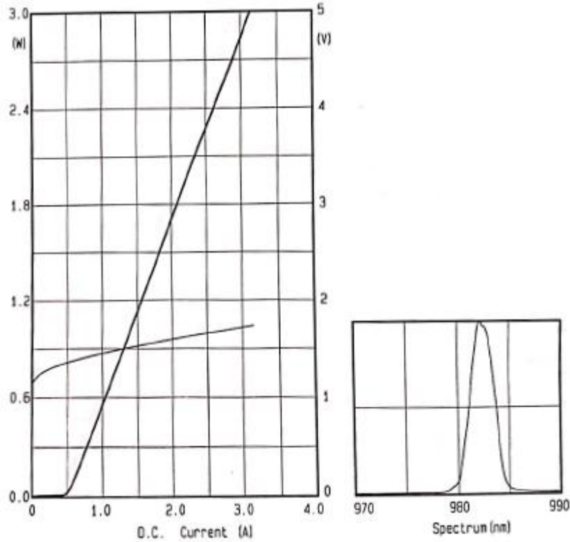
P-I-V 曲线
